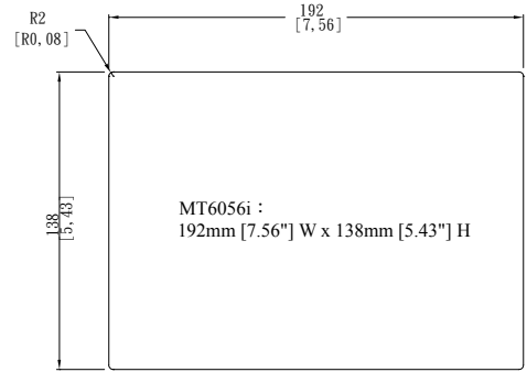
Cutout dimensions
