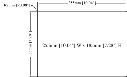
Cutout Dimensions
